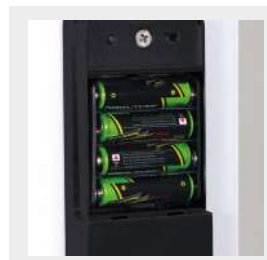
Funciona con 4 pilas alcalinas AA 6V
